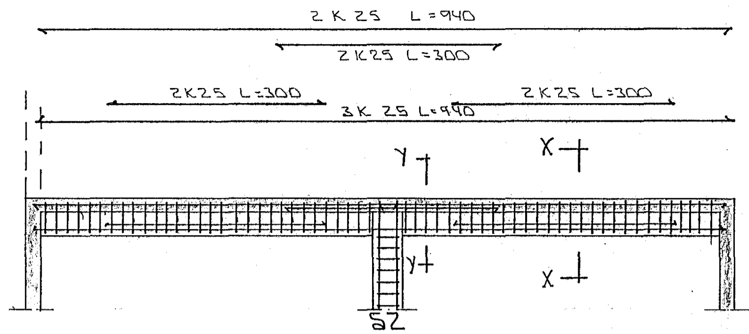
ÁSYND A - A 1:50
