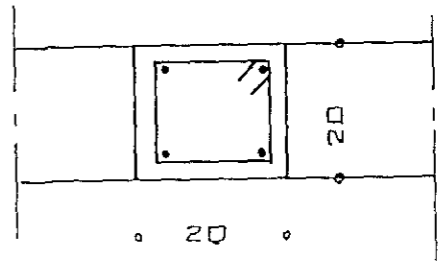
S1 LÖBRET 4 K-12 LARETT LYKKJUR R-10 L=14x14 1/2 20 cm.
