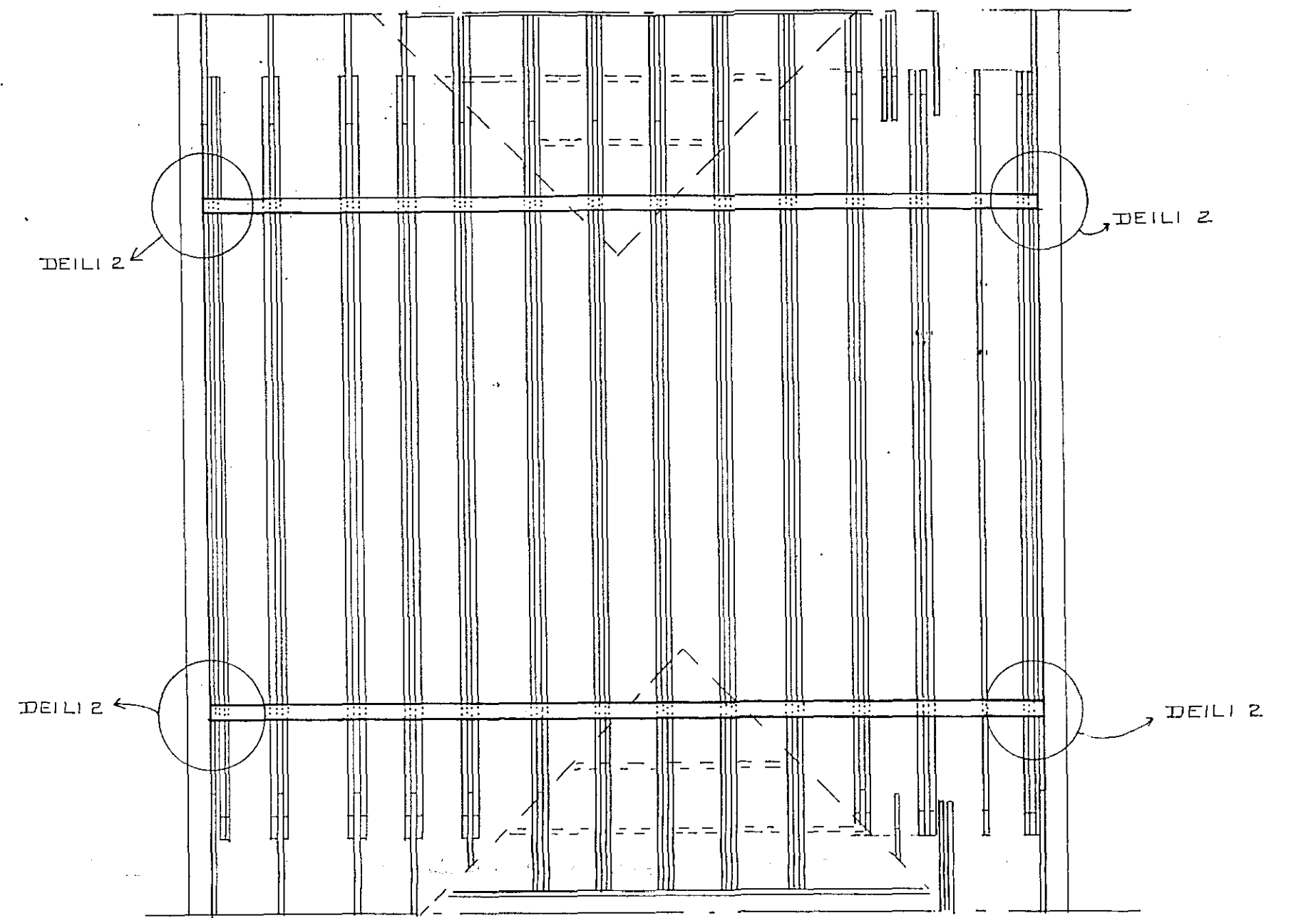
GRUNNMYND GÖLFBITAR.
