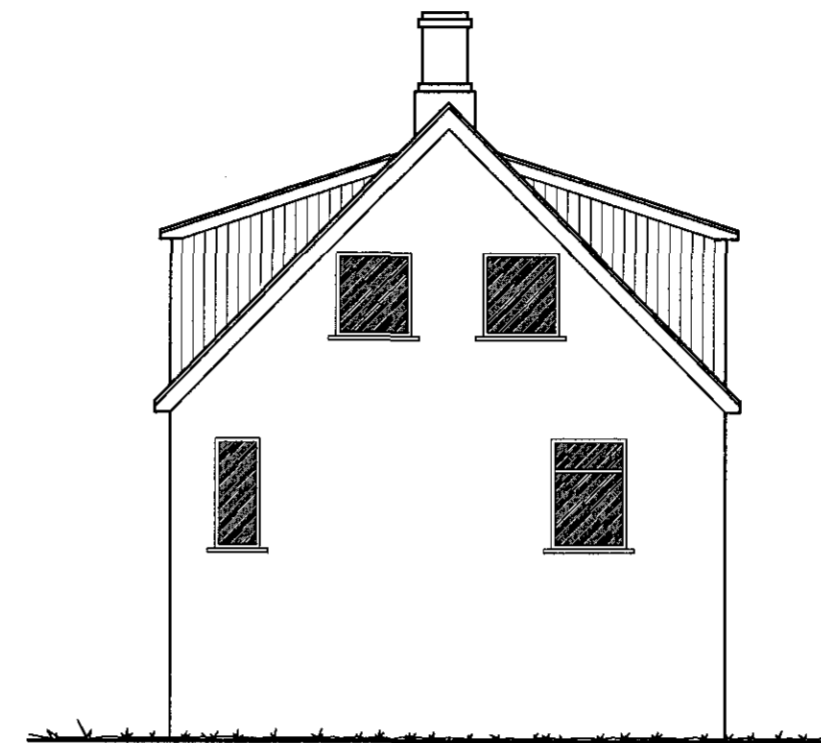
ÚTLIT SUÐUR 1:100
