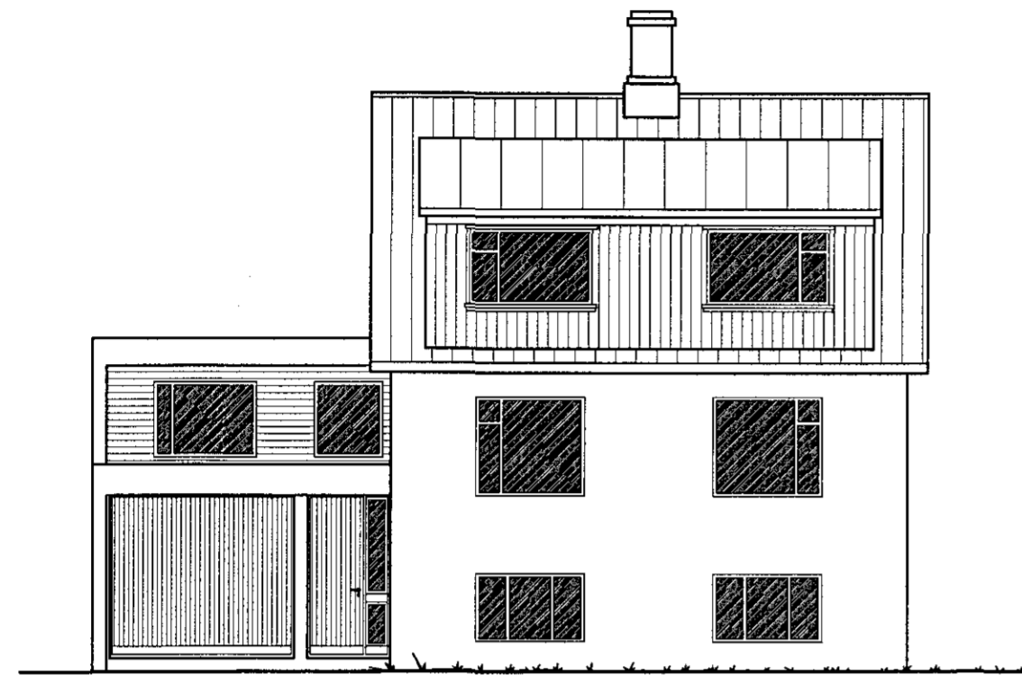
ÚTLIT VESTUR 1:100
