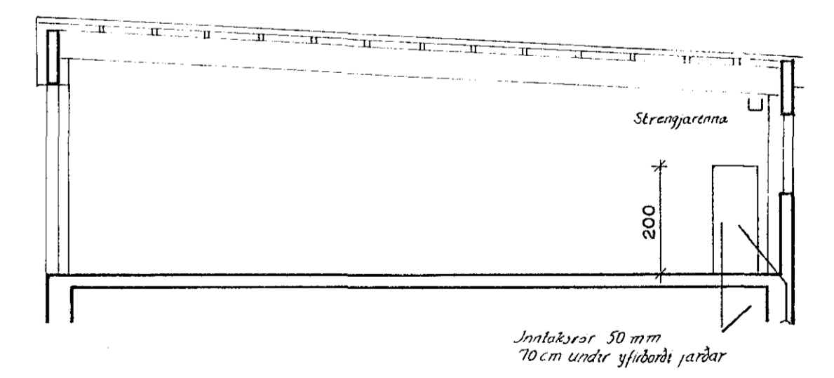
SNID A-A 1:100
