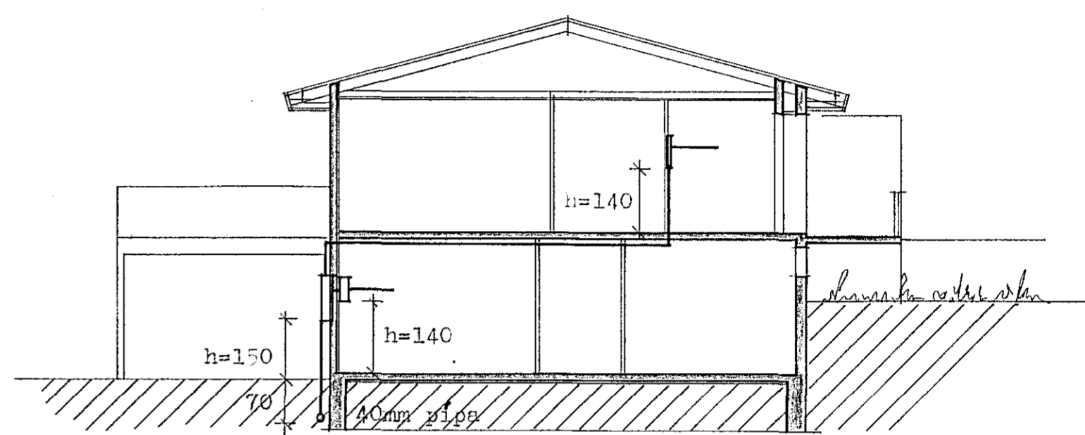
sníð A-A
