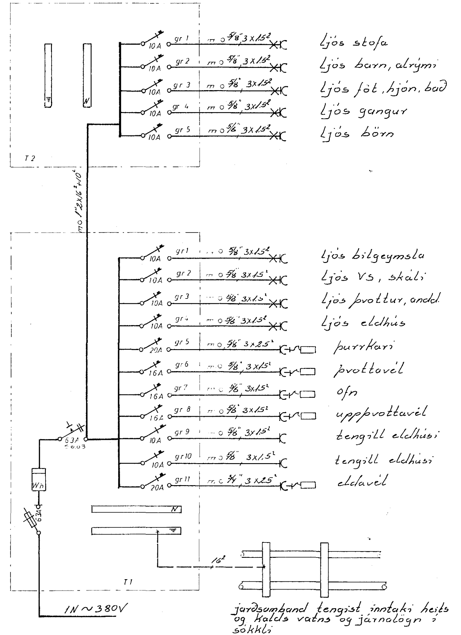
einlinumynd
