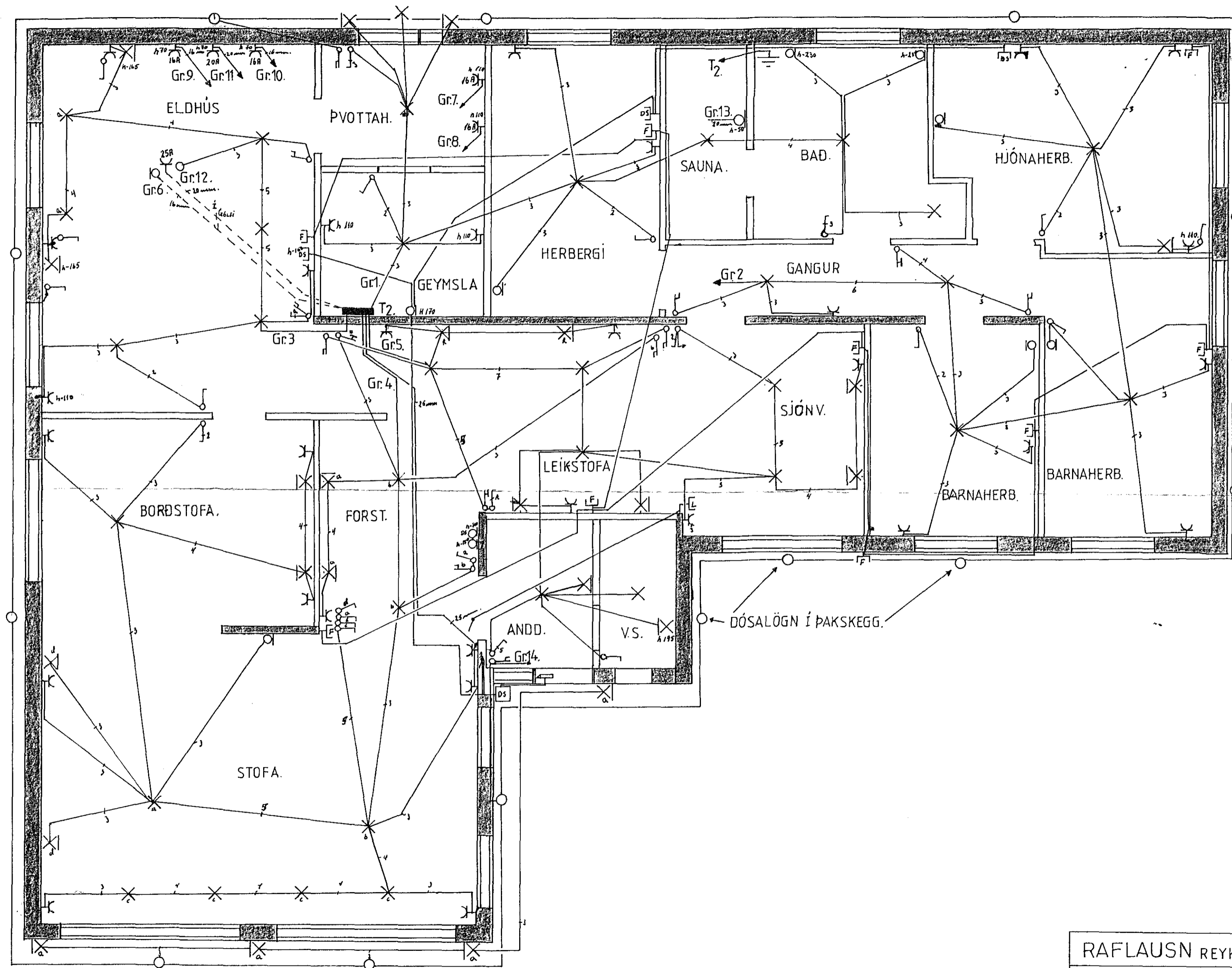
GRUNNMYND RAFLAGNA 1 HÆÐ. 1:50.
