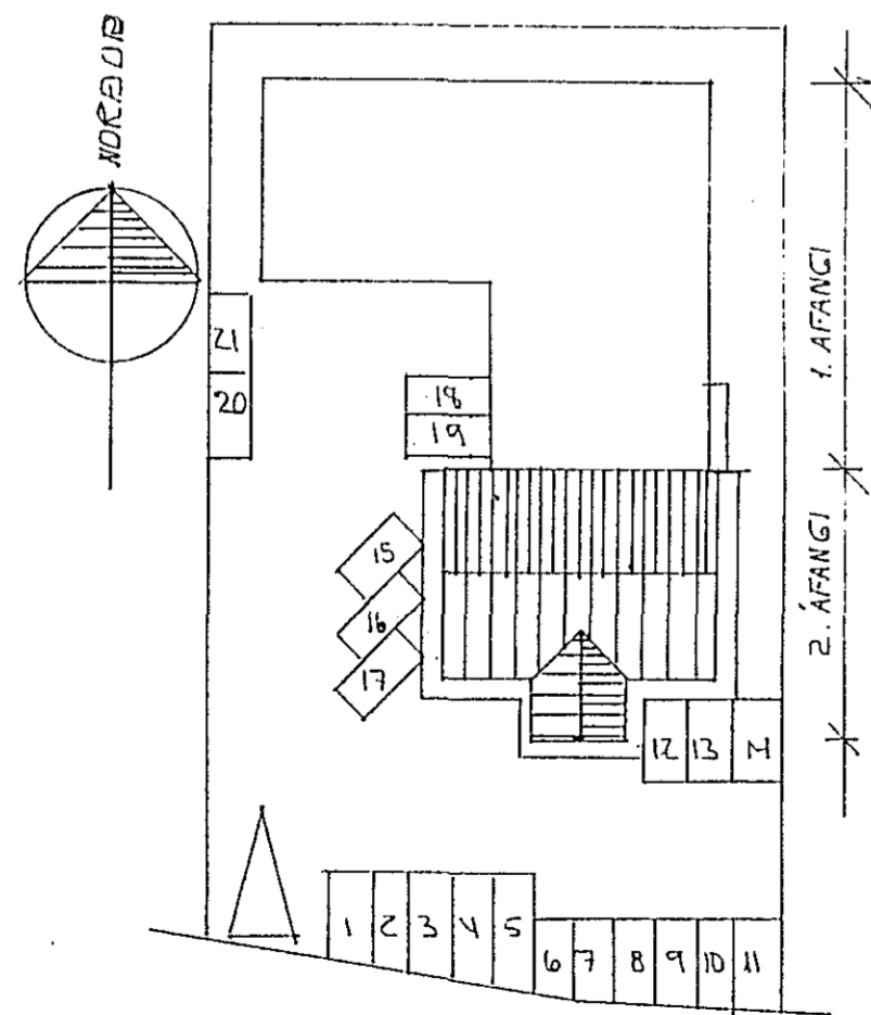
AFSTÖÐUMYND MÆLIKVARÐ 1:500
