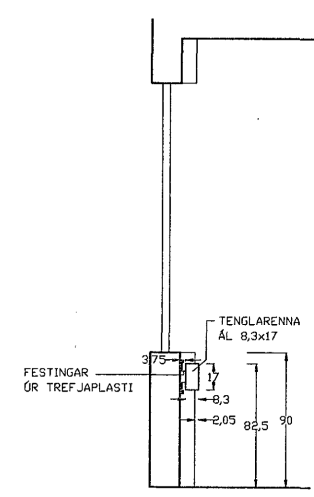
SNID AF FRÁGANGI RENU MÆLIKVARÐI 1:20
