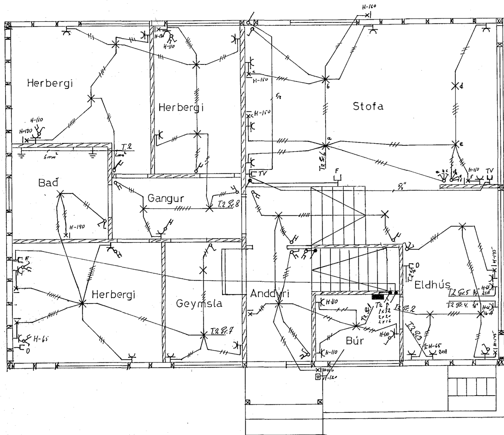
Grunnmynd hæðar 1:50.
