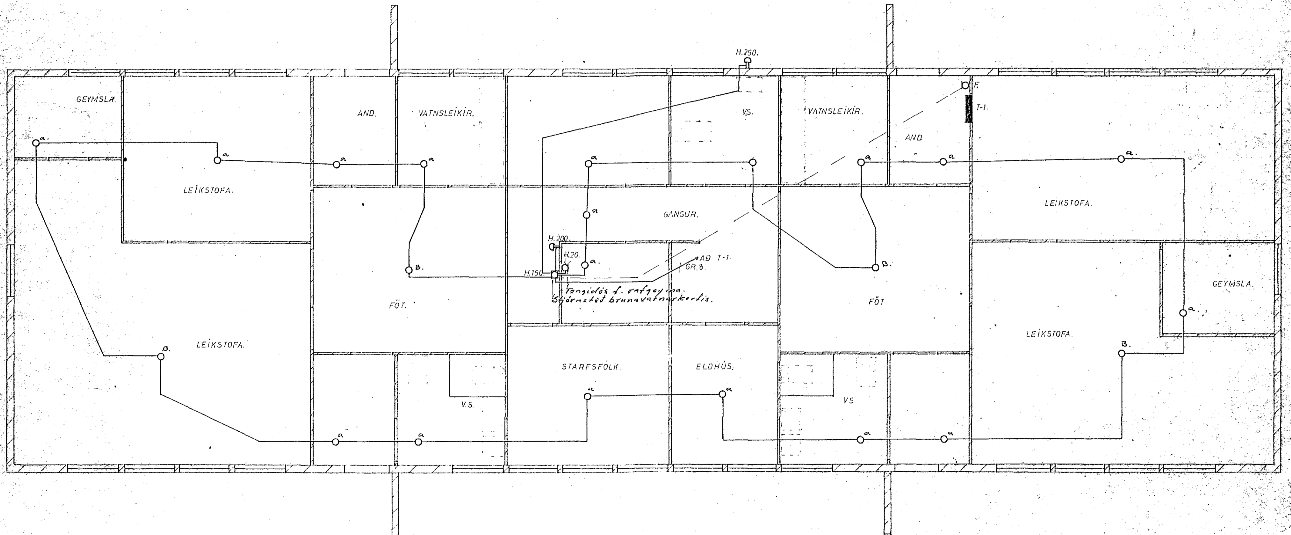
GRUNNMYND 1:50.
