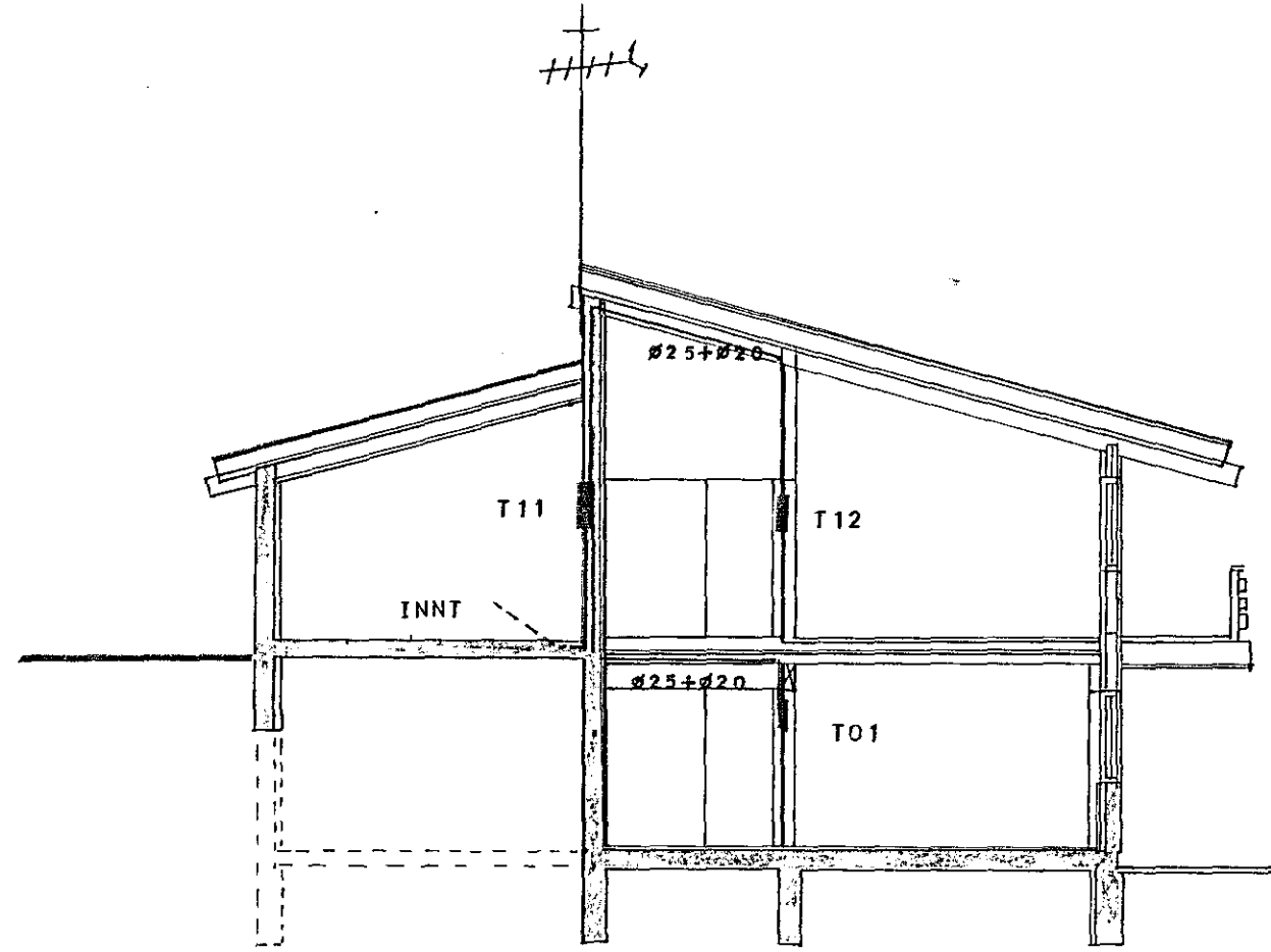
SKURÐUR A-A M 1:100
