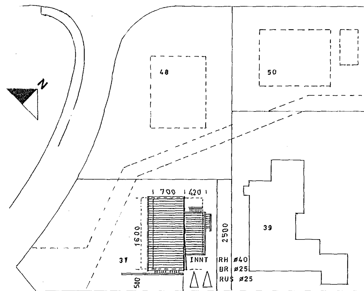
AFSTÖÐUMYND M 1:500 NORÐURBRAUT
