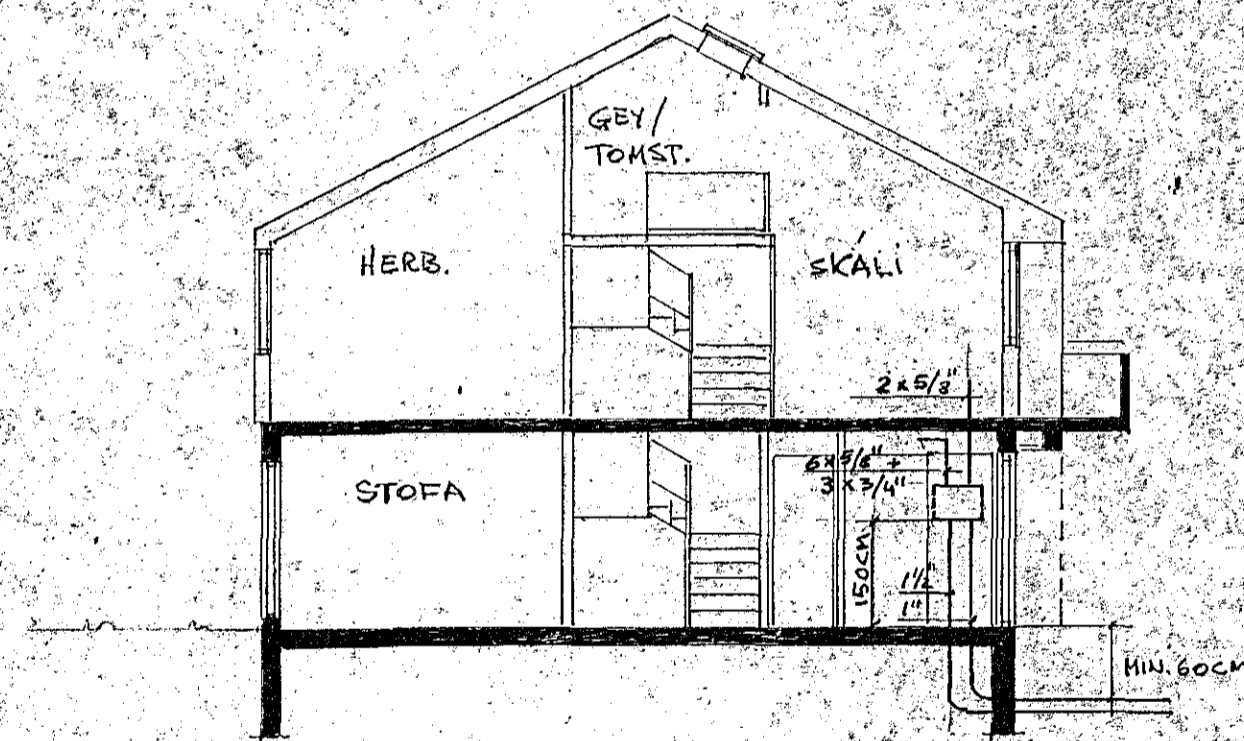
SKURÐUR A-A 1:100
