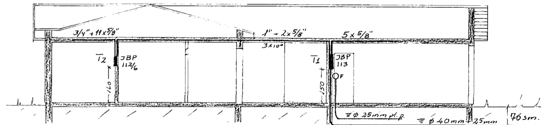
SNID A-A M 1:100
