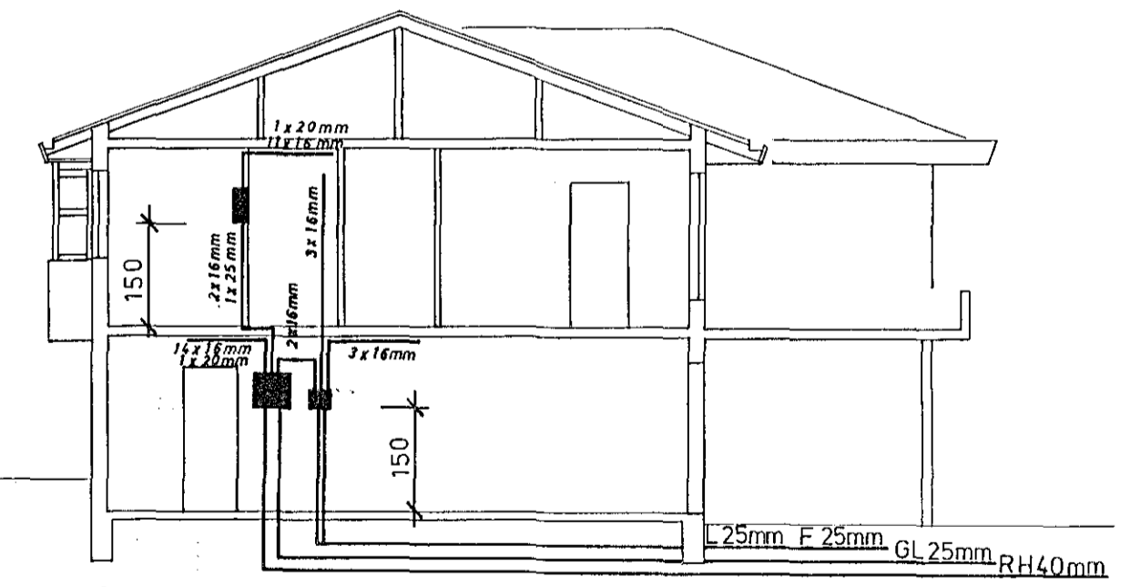
Snid. Mkv. 1:100
