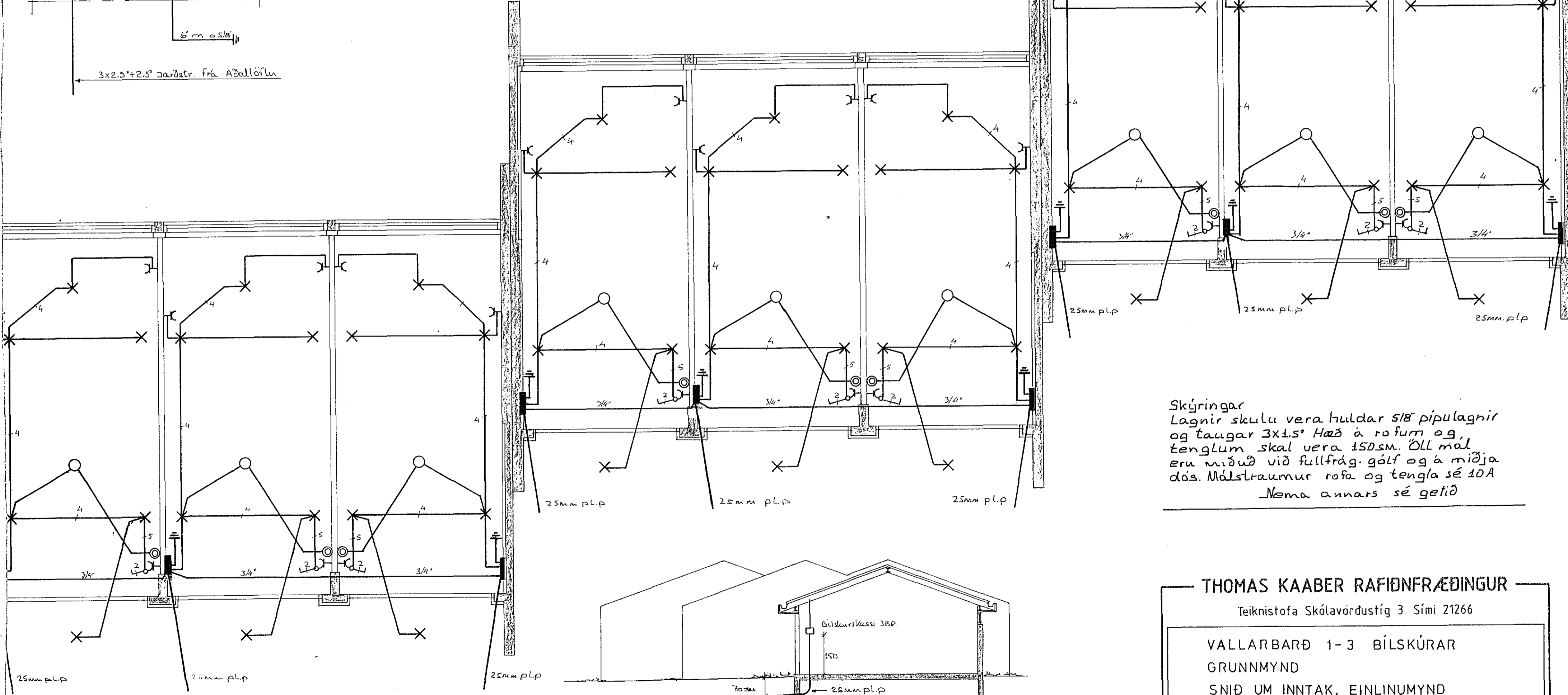
SNÍÐ UM INNTAK M=1:100
