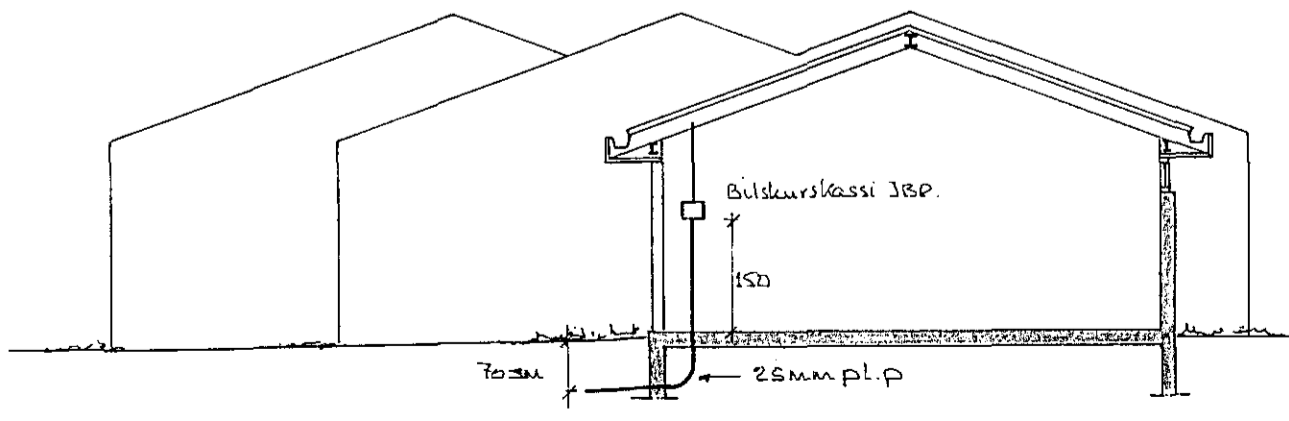
SNÍÐ UM INNTAK M=1:100
