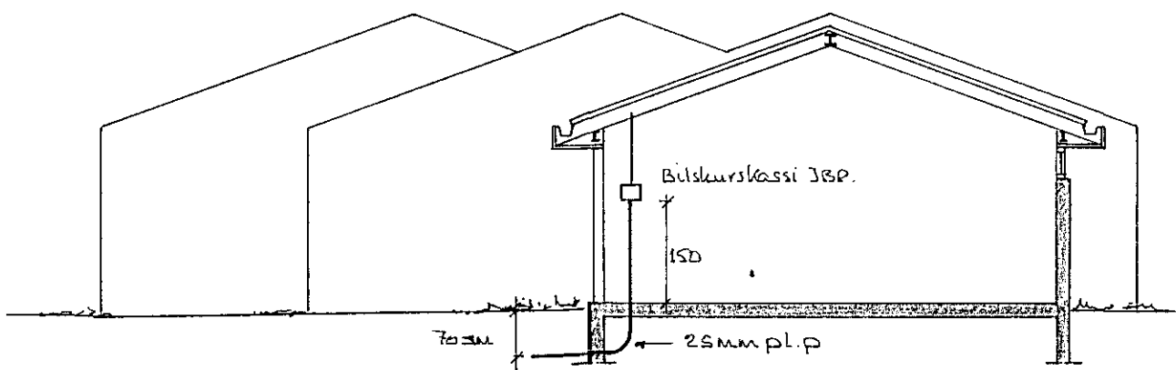
SNÍÐ UM INNTAK M=1:100
