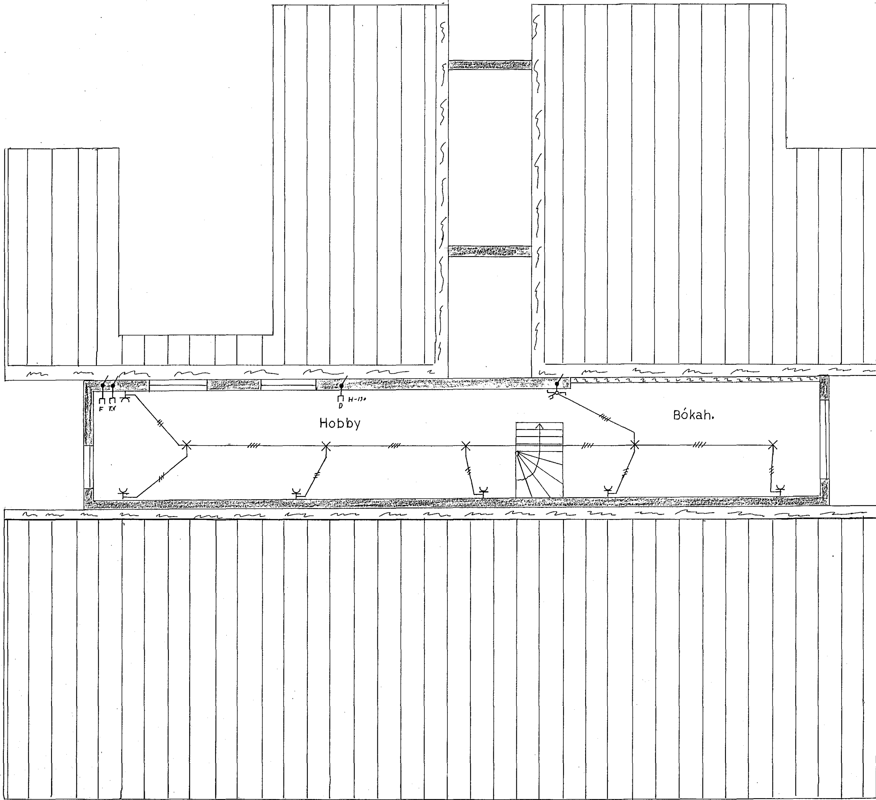
Grunnmynd ris. 1:50
