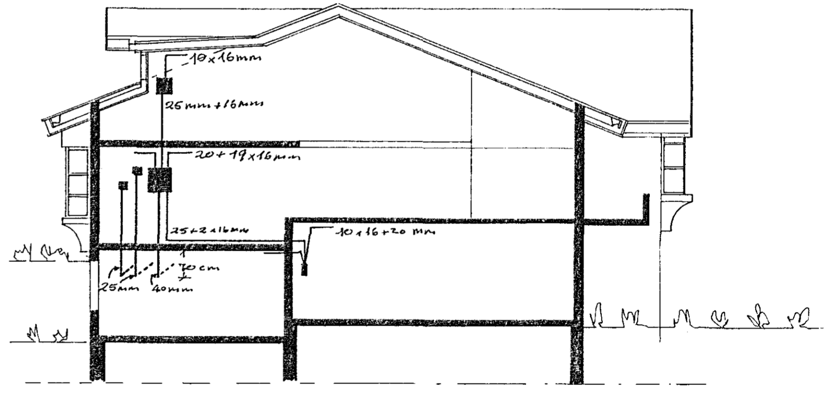
SKURÐUR.
