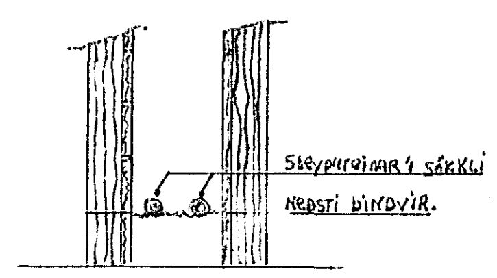
SNID A-A Í GRUNNVEGG
