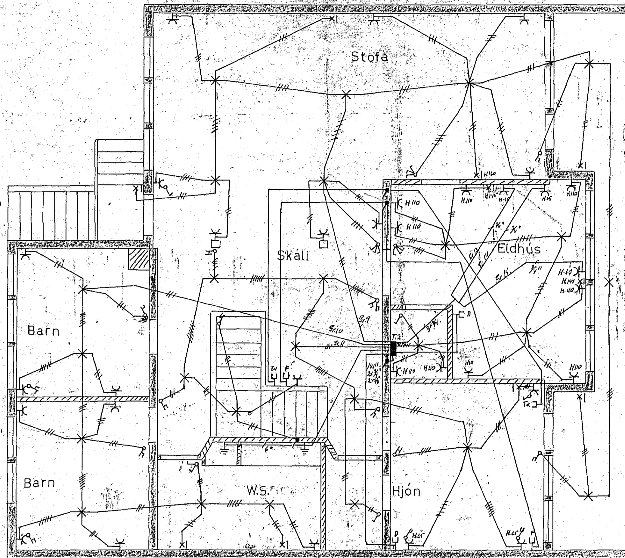
Grunnmynd 2 Hæð 1:50
