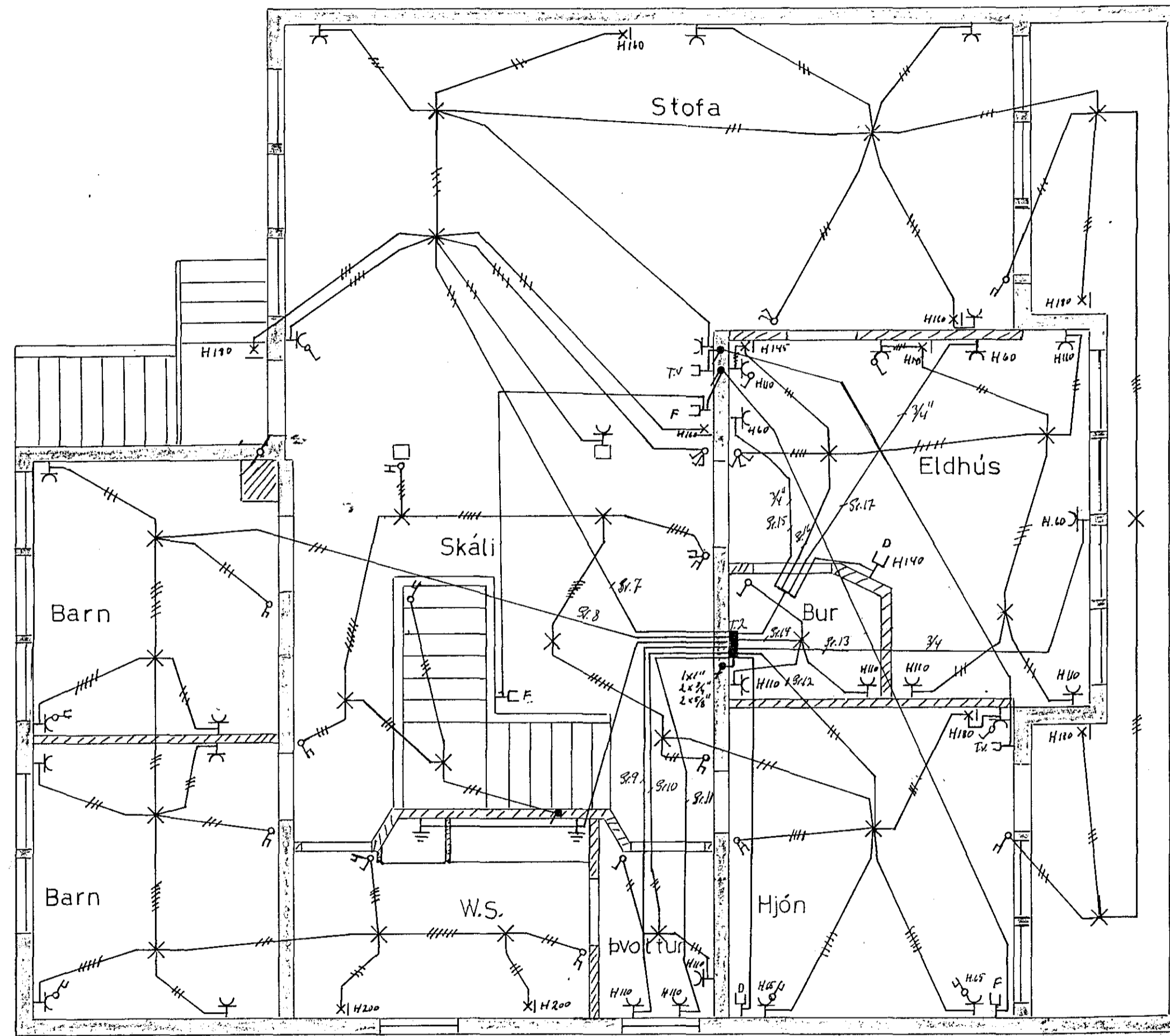
Grunnmynd, 2. hæð 1:50
