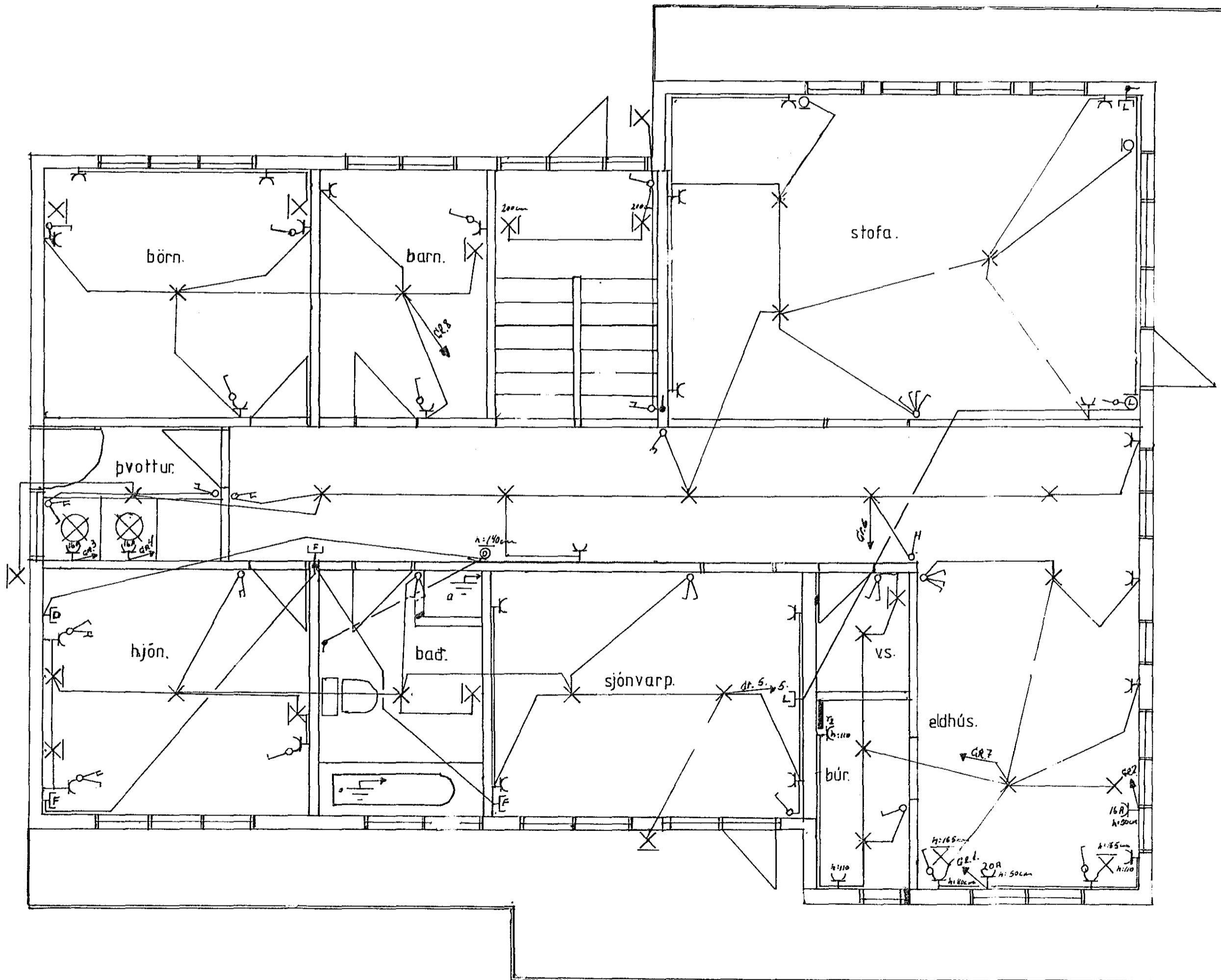
GRUNNMYND 2.HÆÐ. 1:50
