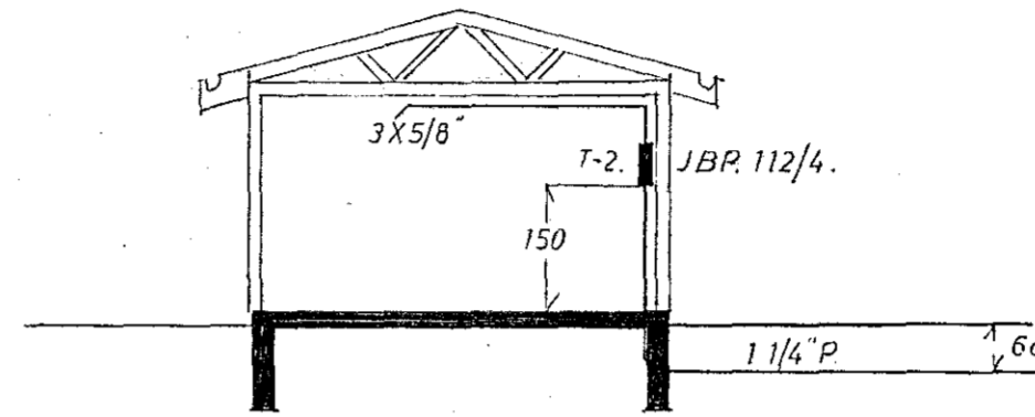
SNÍÐ BÍLSKÚR 1:100.
