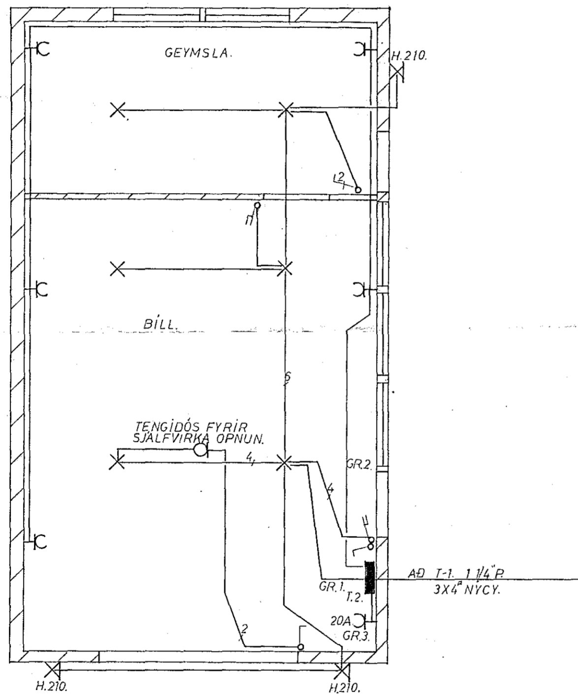
GRUNNMYND BÍLSKÚR 1:50.
