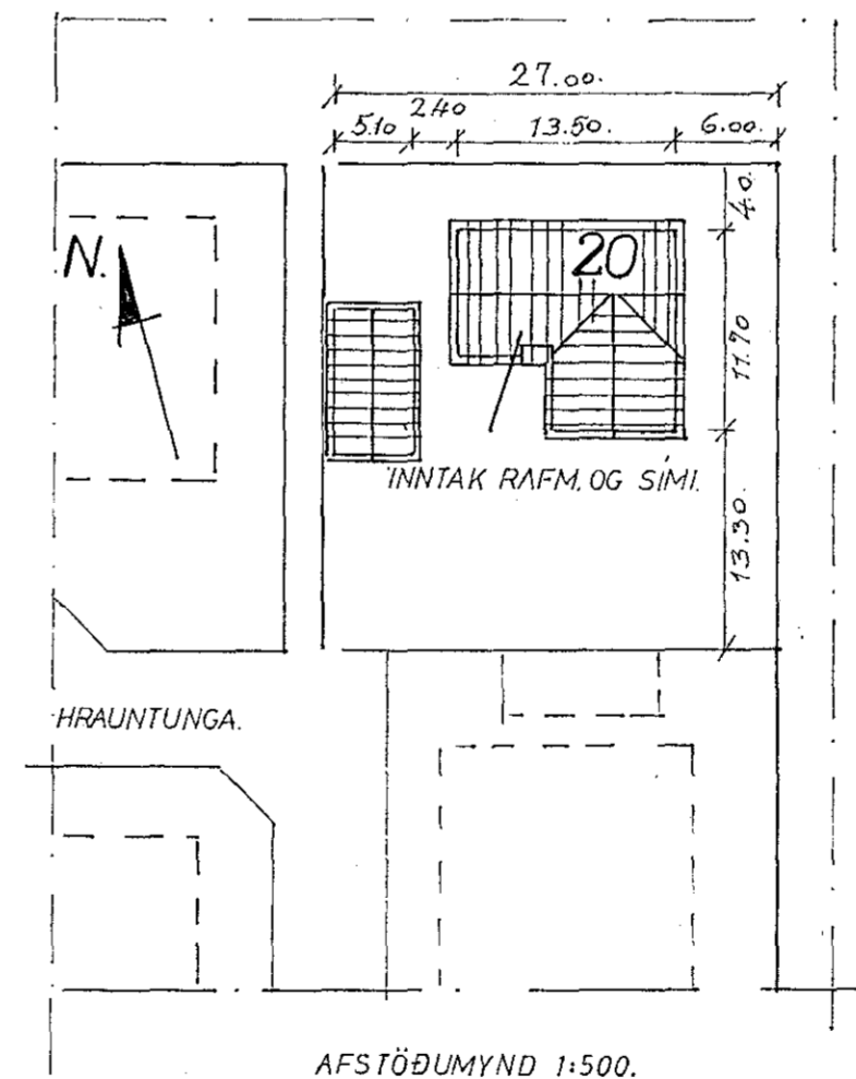
AFSTÖÐUMYND 1:500.
