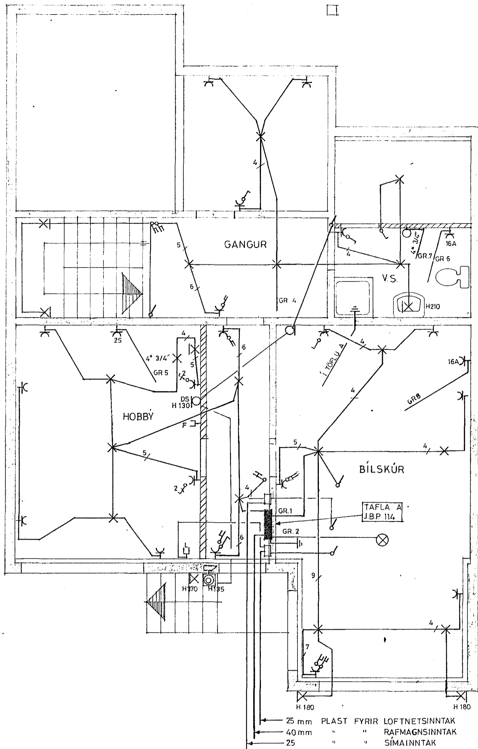
GRUNNMYND KJALLARA 1:50
