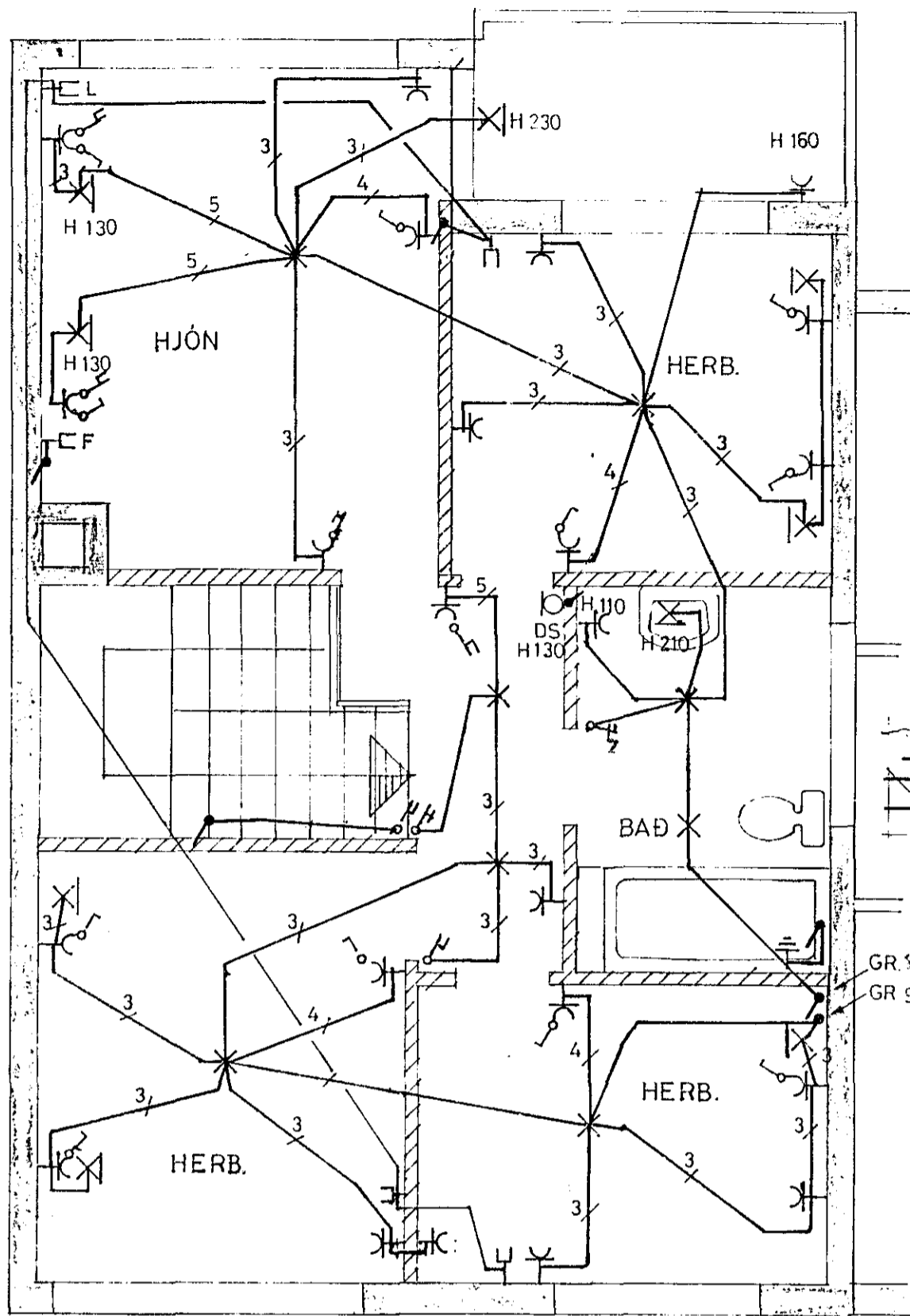
GRUNNMYND 2. HÆÐAR 1:50
