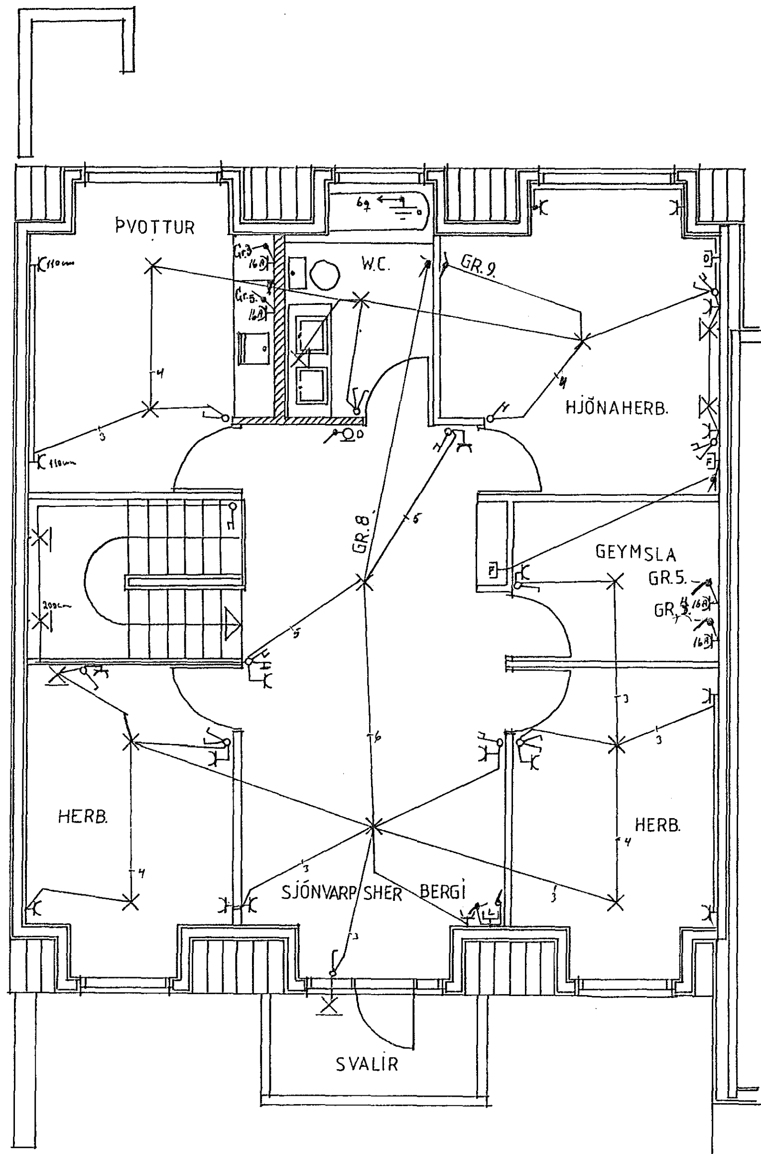
2. HÆÐ. GRUNNMYND. 1:50
