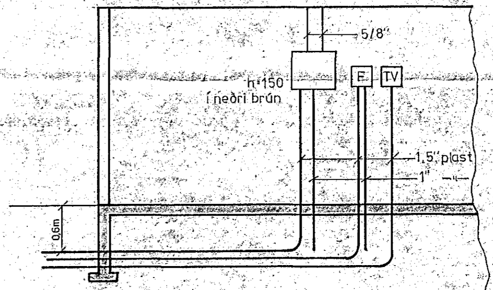
Snið A-A
