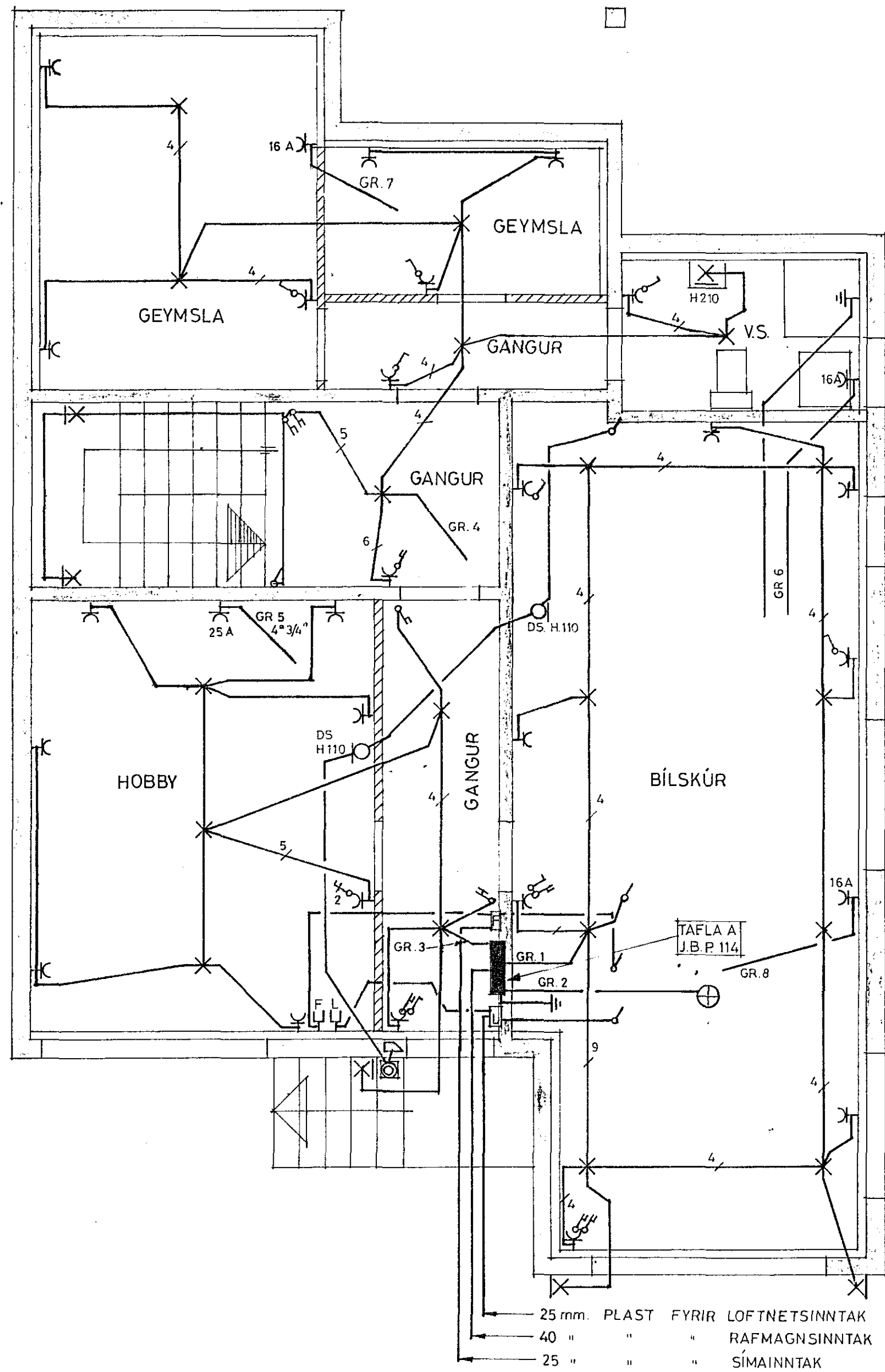
GRUNNMYND KJALLARA 1:50
