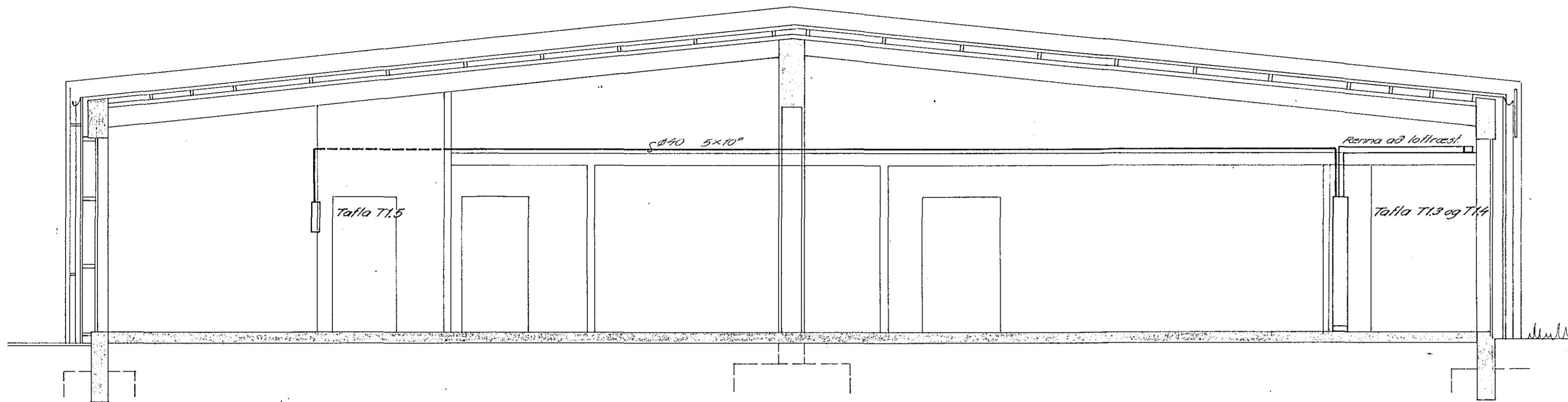
I-V Þversnið M=1:50
