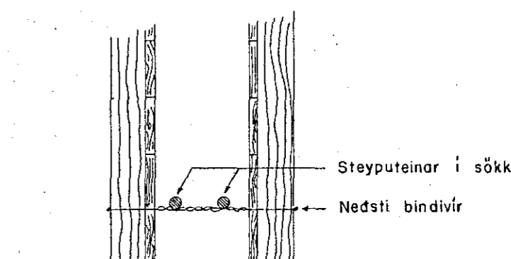
SNÍÐ B-B Í GRUNNVEGG
