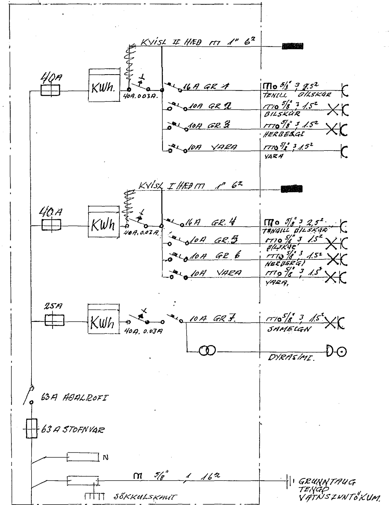
ADALTAFLA EINLÍNEMYND.
