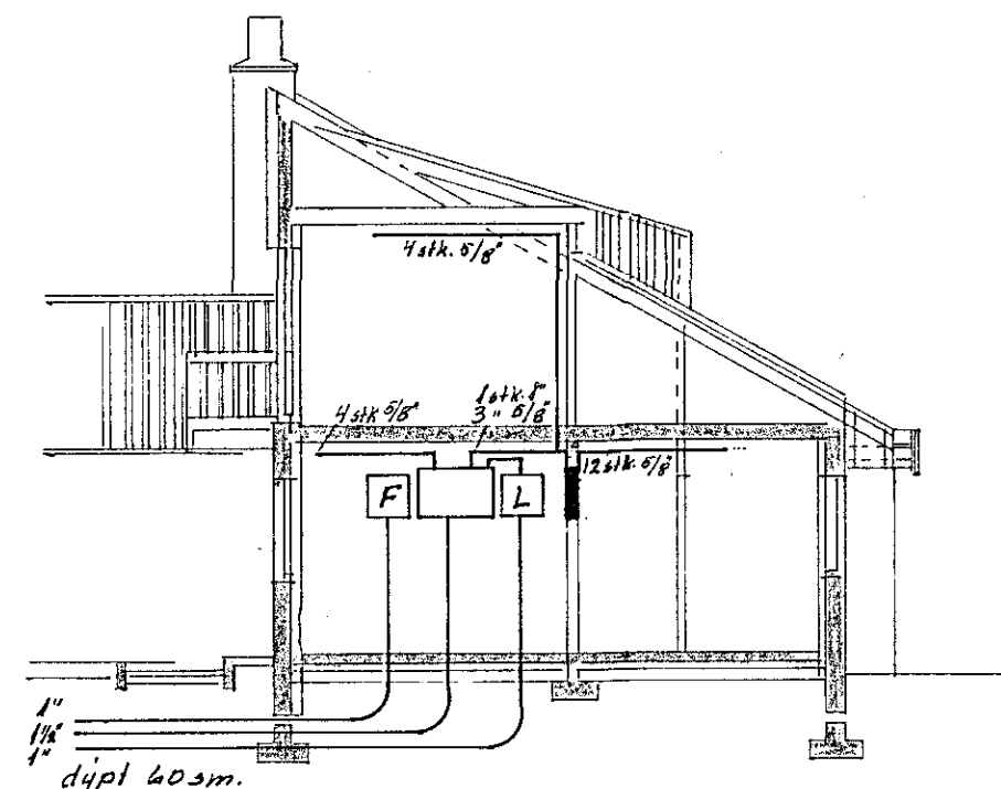
Skurður 1:100
