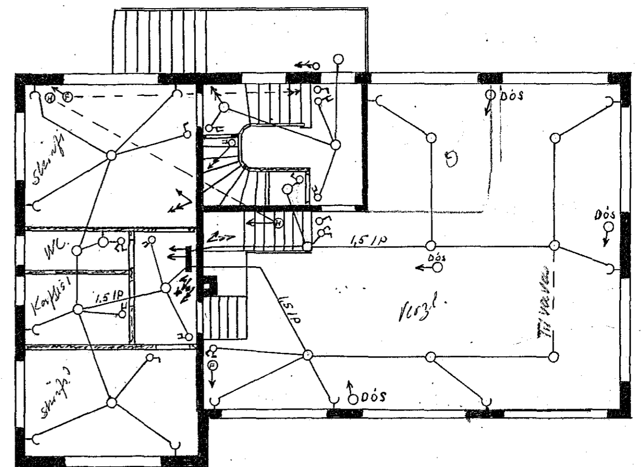
2. hæð
