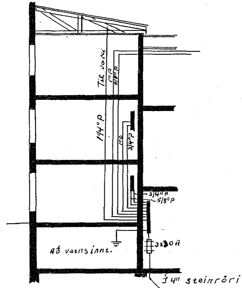
Þverskurður
