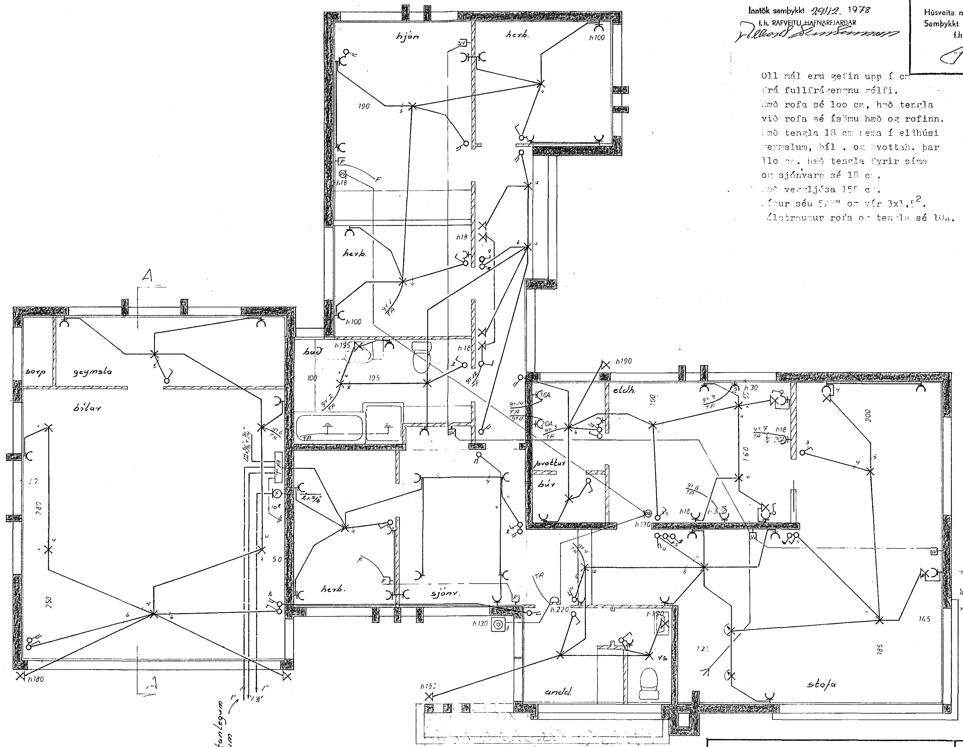
grunnmynd
