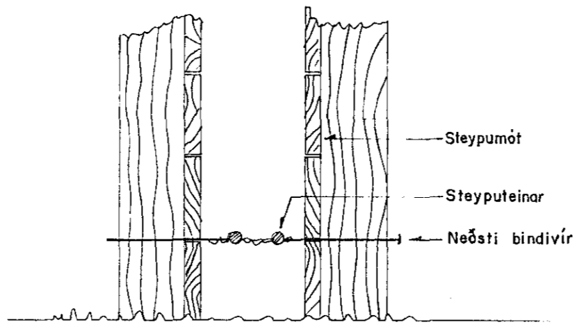
SNIÐ A-A Í STEYPUMÓT
