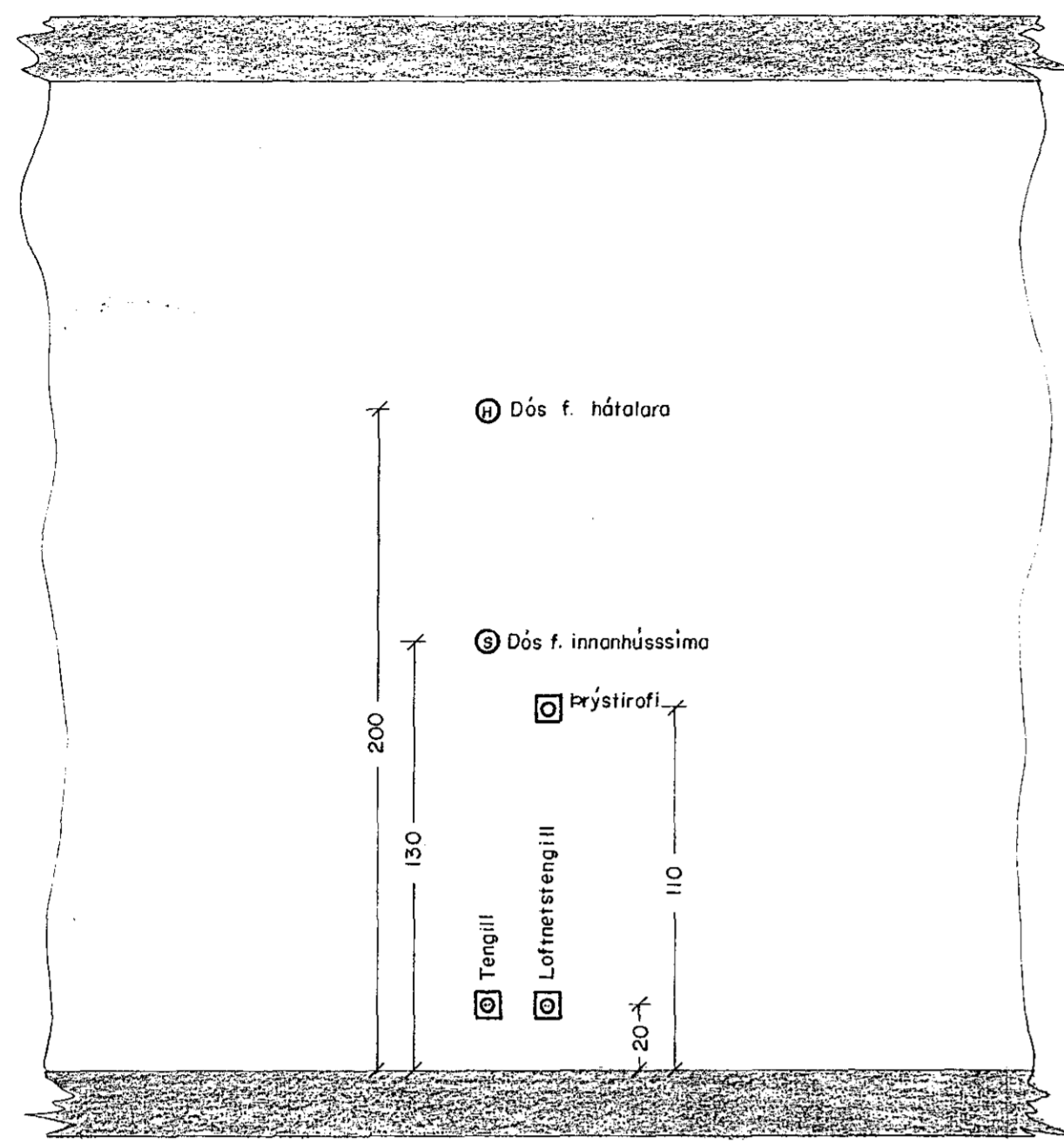
SNID C-C, M=1:20. SJÁ BL. 4 OG 7
