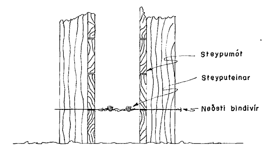
SNID D-D Í STEYPUMÓT.
