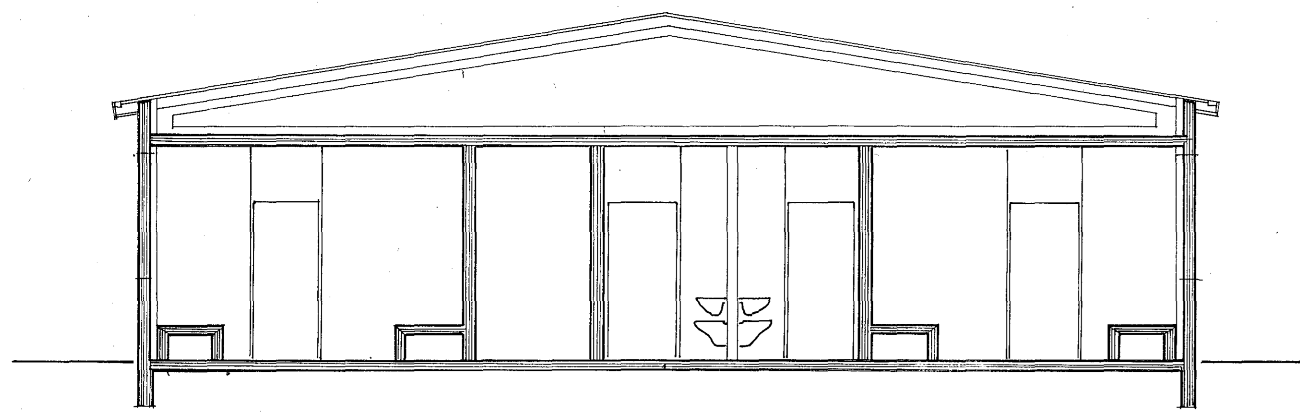
SNEIBING Í KLEFA 1:50
