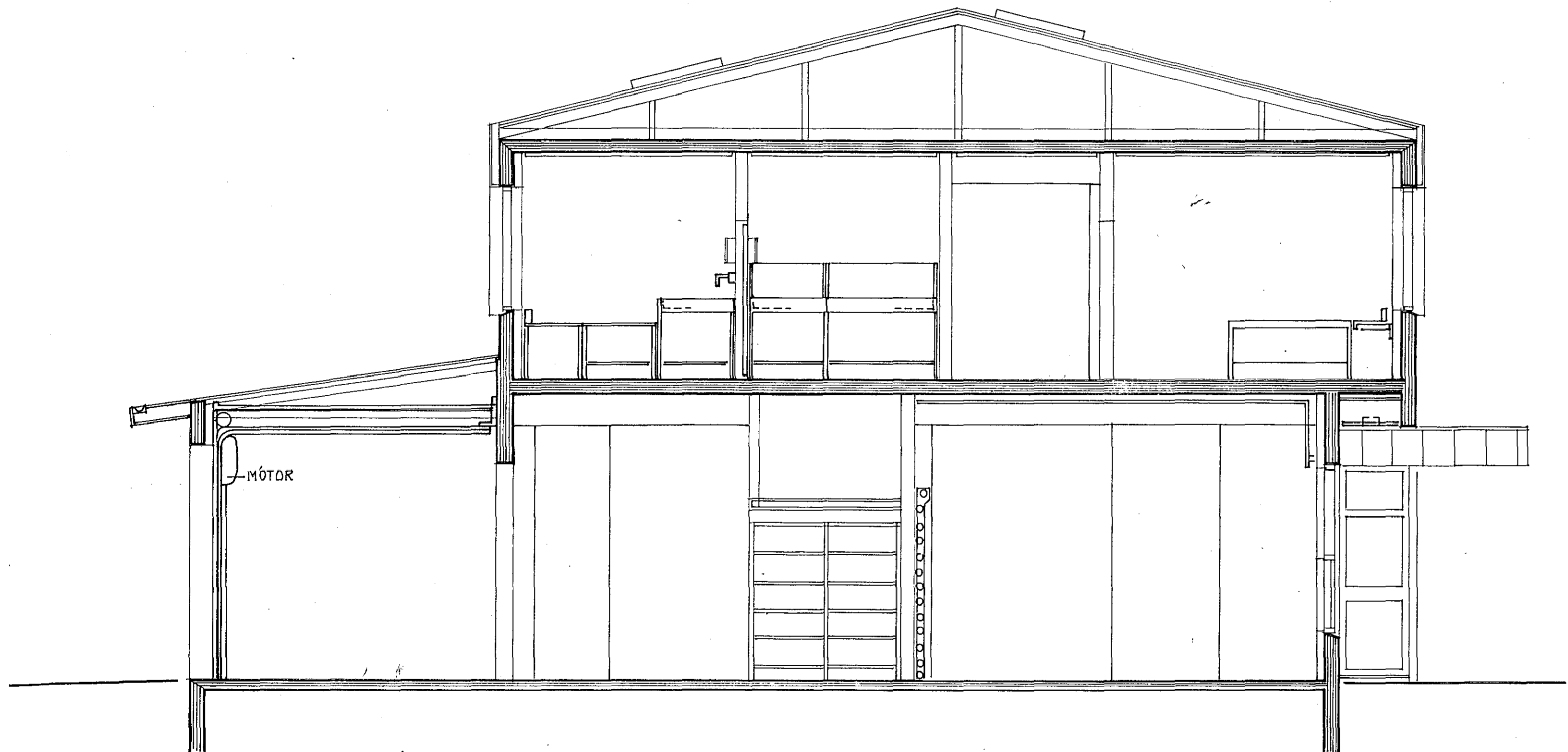
SNEIBING Í SUÐURHLUTA 1:50
