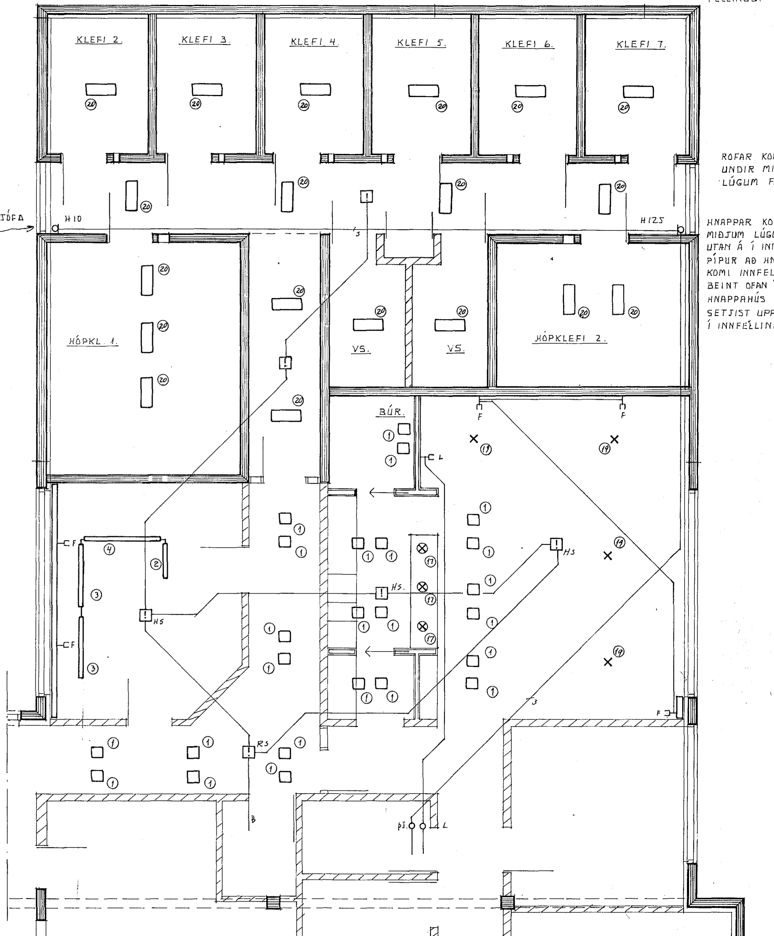
TÖLUR Í HRING VIÐ LAMPA MERKIR NR. LAMPA SAMKV. LAMPASKRÁ
