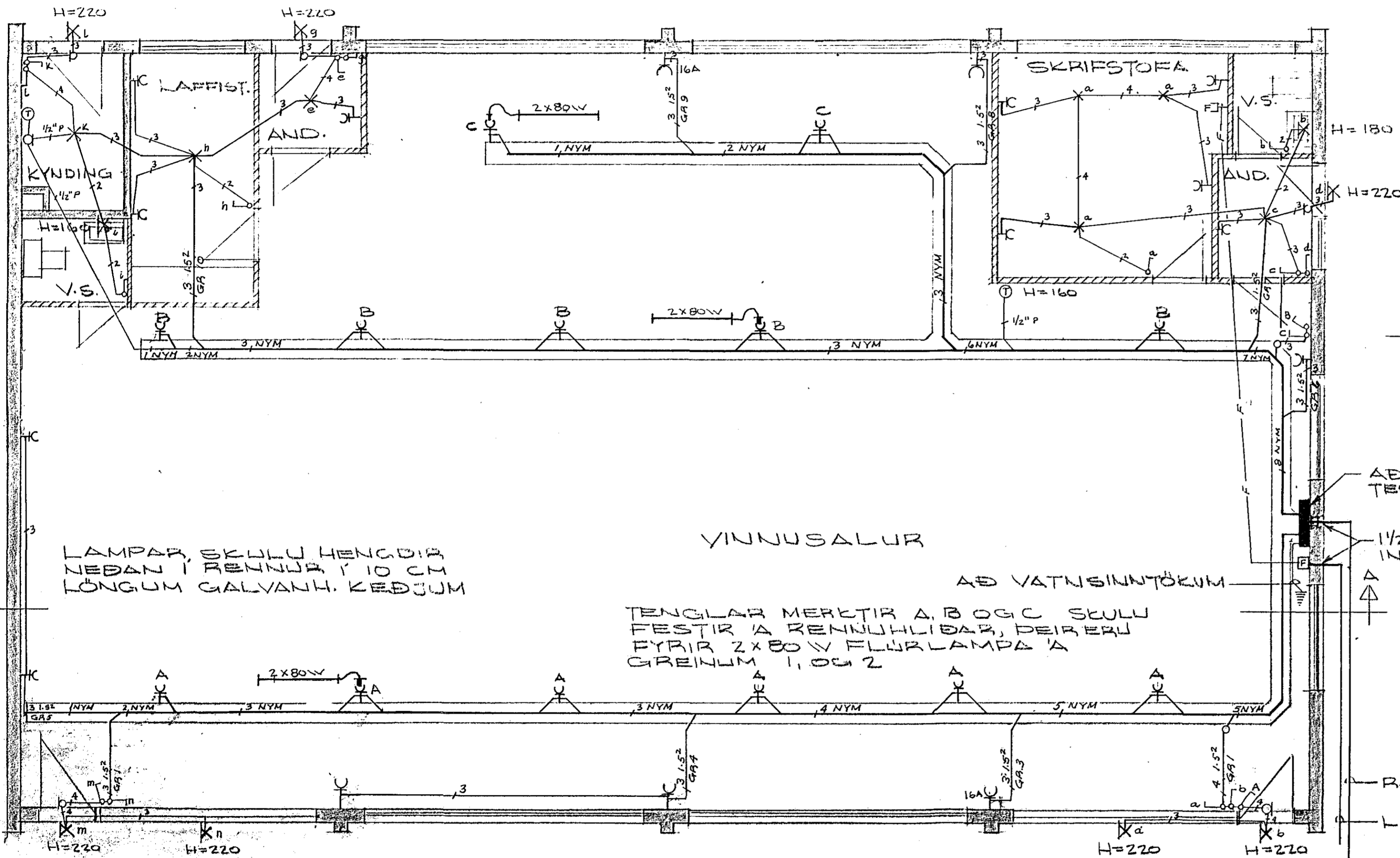
GRUNNMYND KYRÐI 1:50
