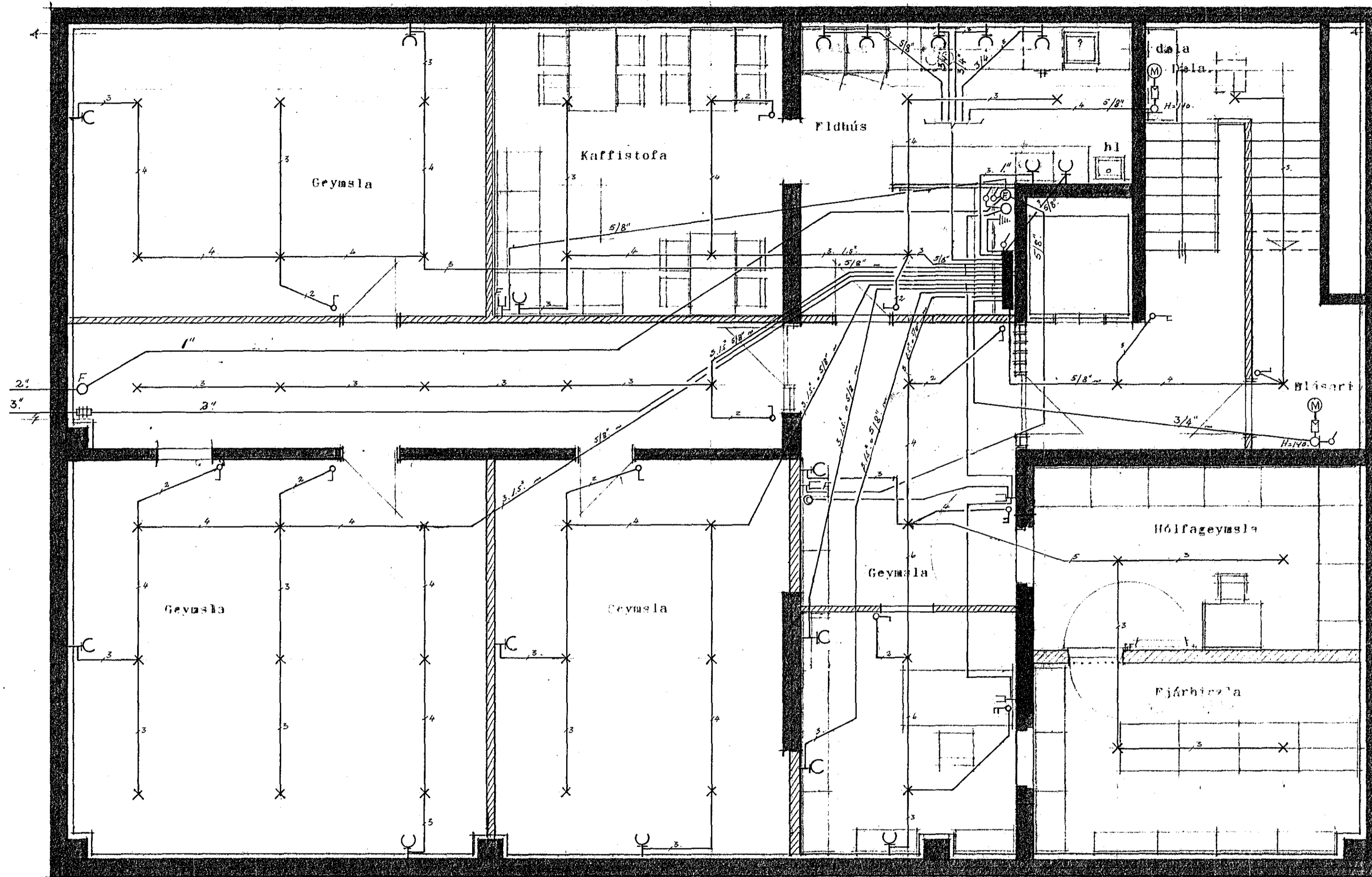
grunnmynd kjallara
