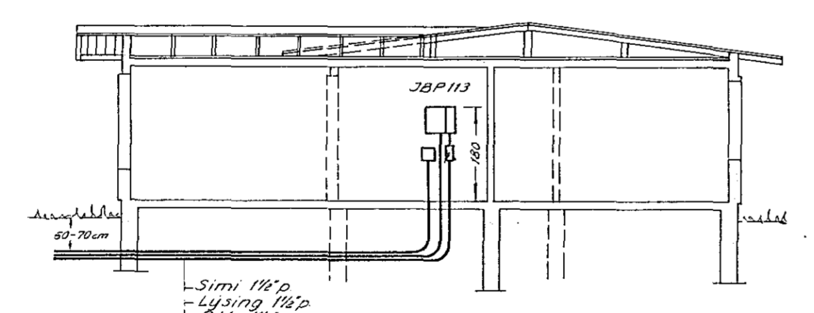
BVERSNIÐ B-B M=1:100
