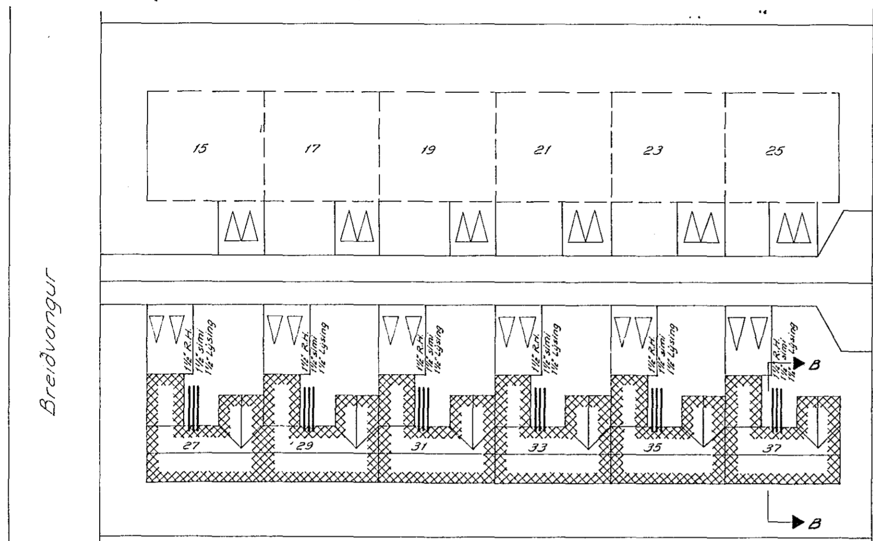
AFSTÖÐUMYND M=1:500
