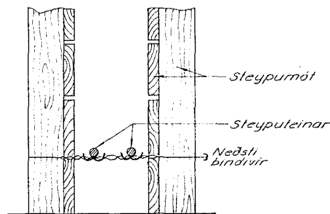
Snið í sökkul
