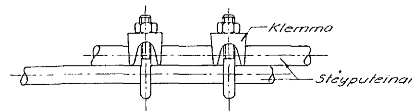
Samtenging teina allan hringinn í sökklinum
