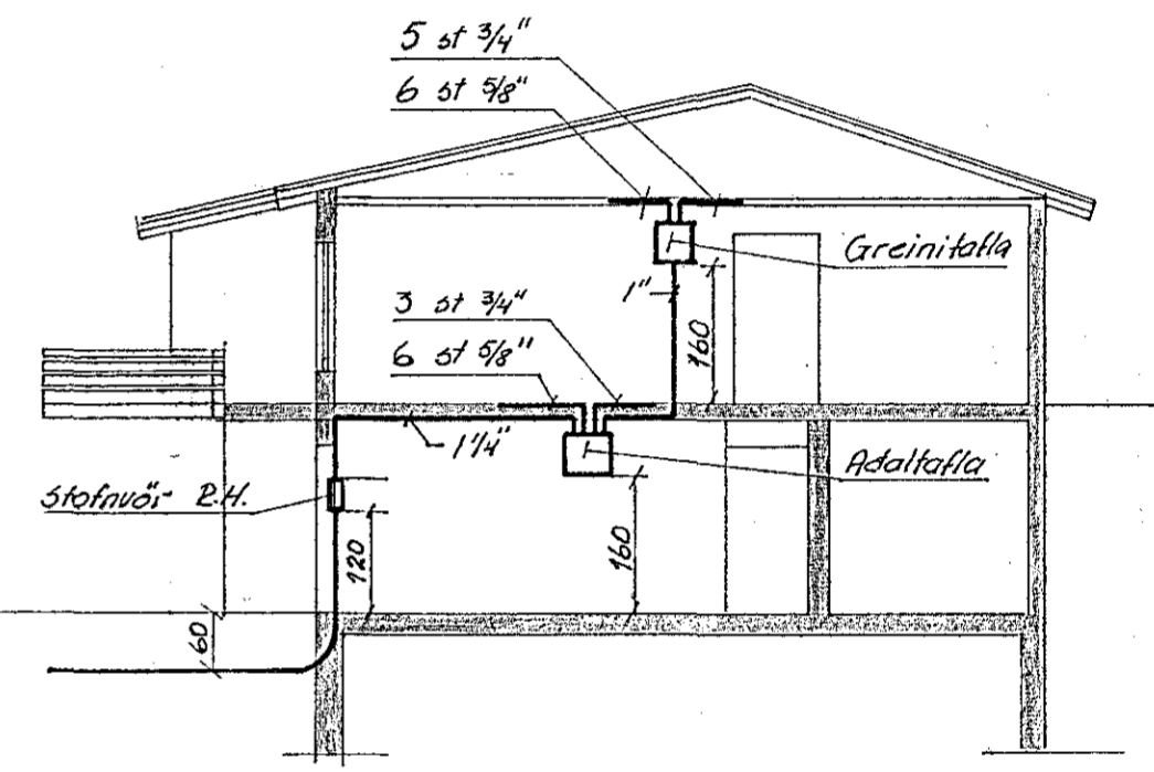
SNID A-A 1:100
