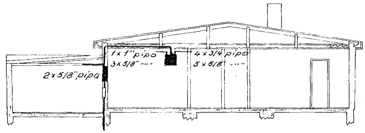
Þversnið
