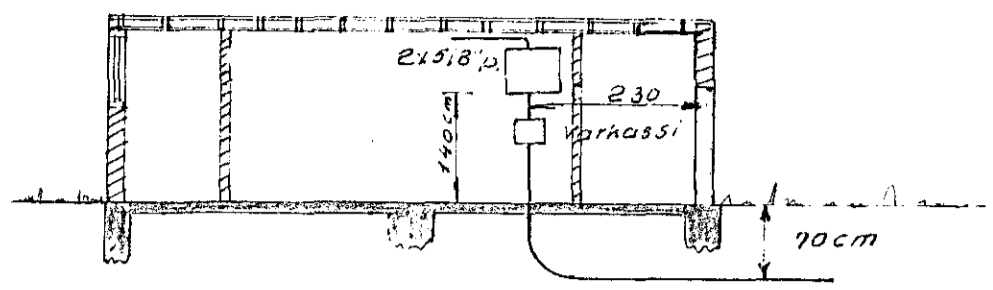
Bilgeymsla, þverskurður sem sýnir staðsetn. töflu.
