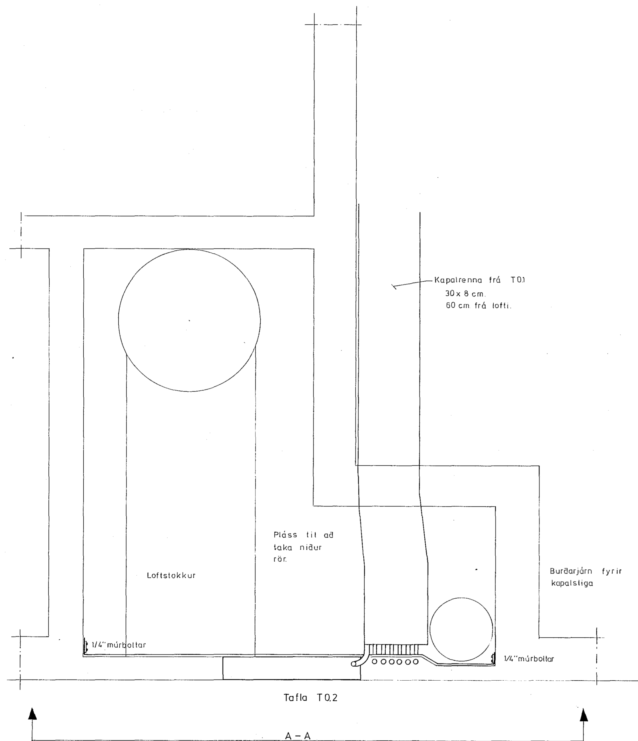
Grunnmynd M.1:10
