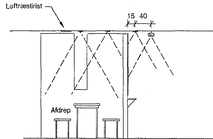
MKV 1 : 50 Sneiding A - A
