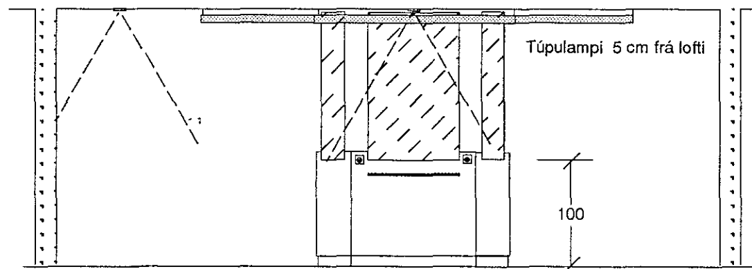
MKV 1 : 50 Sneiding B - B
