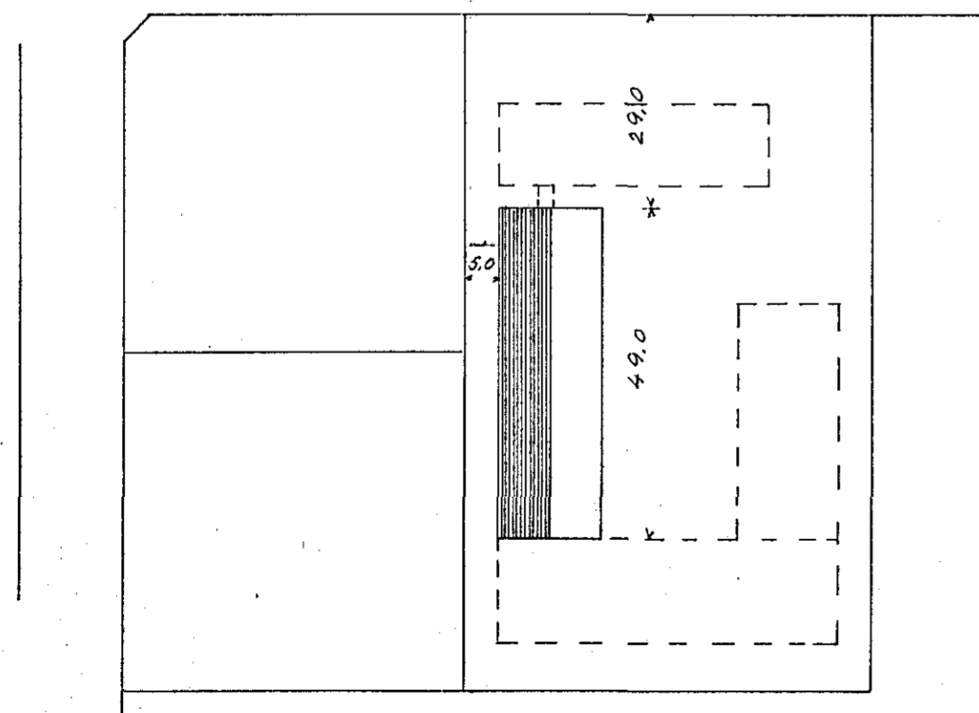
AFSTÖÐUMYND 1:1000
