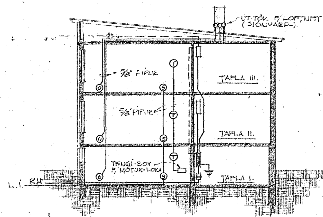
SKURUR MÁL 1100
